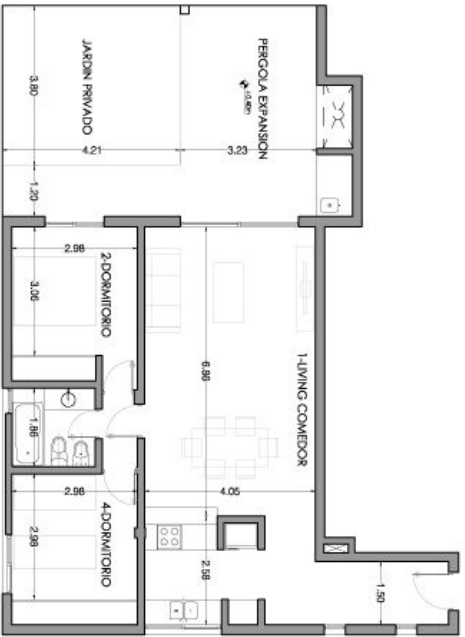
UNIDAD 'A' - PLANTA BAJA - 83 m 2 CUBIERTOS + 21 m 2 SEMICUBIERTOS
