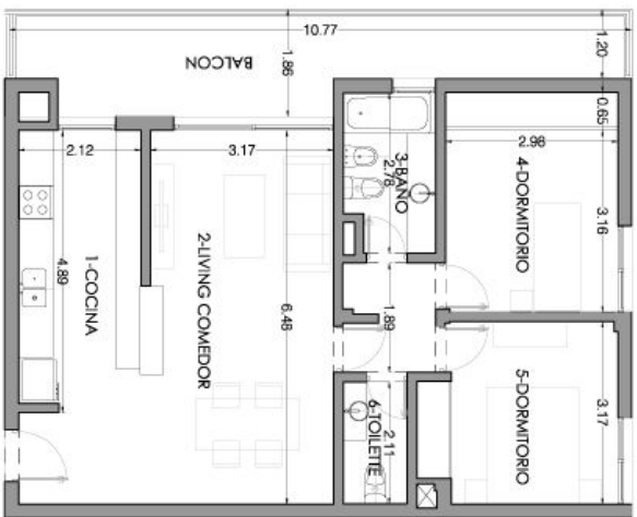
UNIDAD "D" PLANTA TIPO - 77,5 m 2 CUBIERTOS + 16 m 2 BALCON
