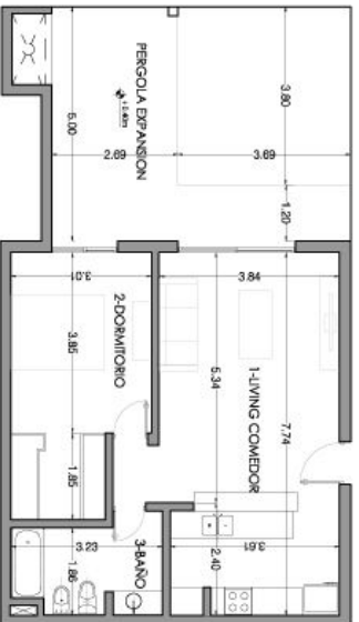
UNIDAD 'B' - PLANTA BAJA - 63 m 2 CUBIERTOS + 17 m 2 SEMICUBIERTOS
